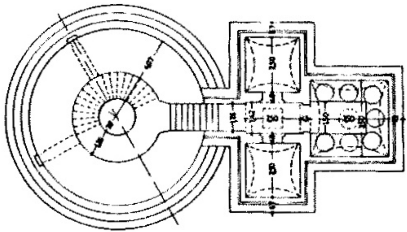
Grundriß des Ölkellers
