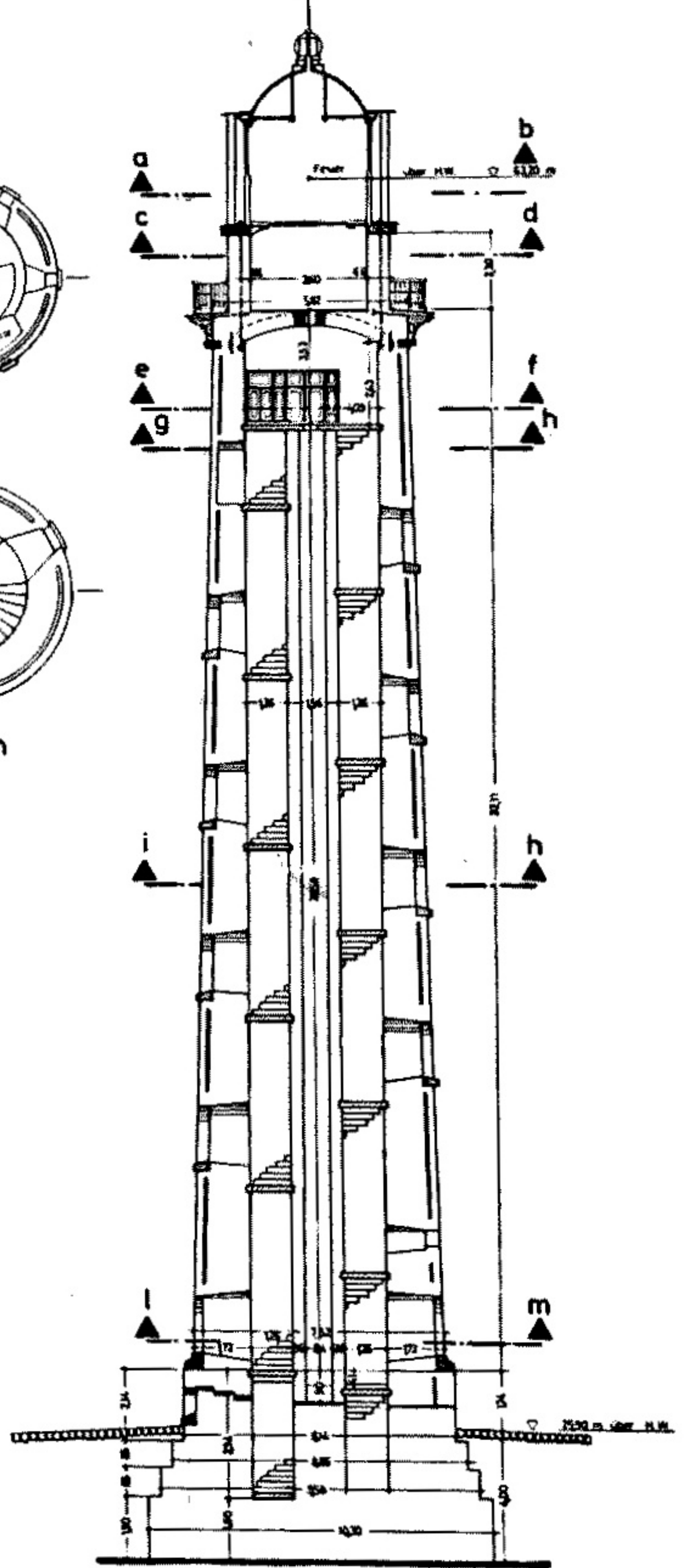
Verticalschnitt
